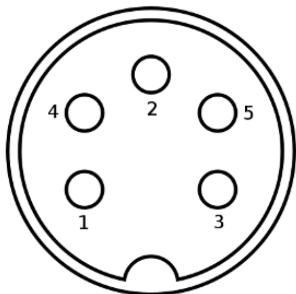
prise DIN vue de face à l'arrière du décodeur
